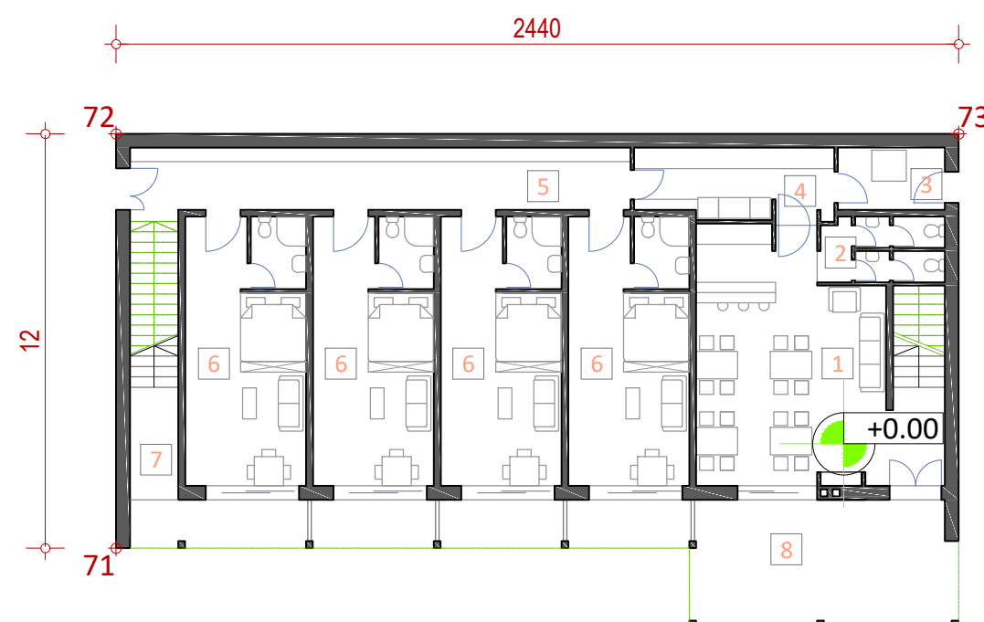
OSNOVA PRIZEMLJA
