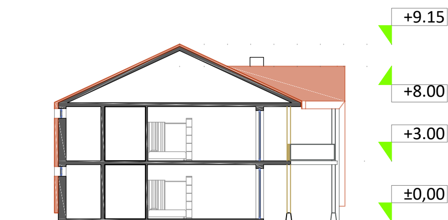
POPREČNI PRESEK
