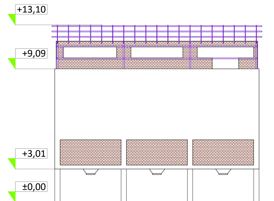
FRONTALNA FASADA
