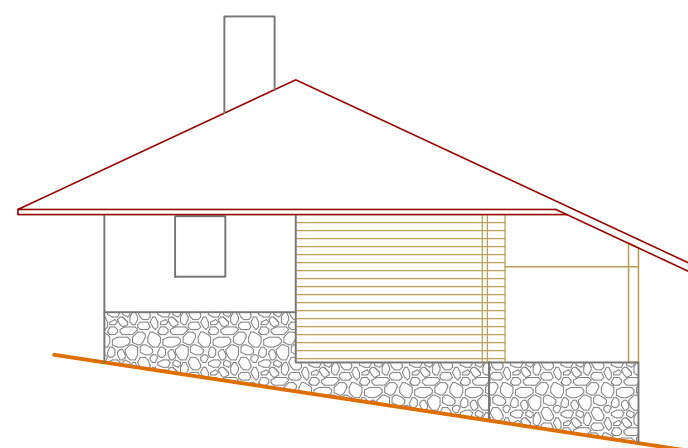
BOČNA FASADA
