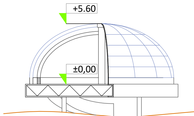
PRESEK / IZGLED
