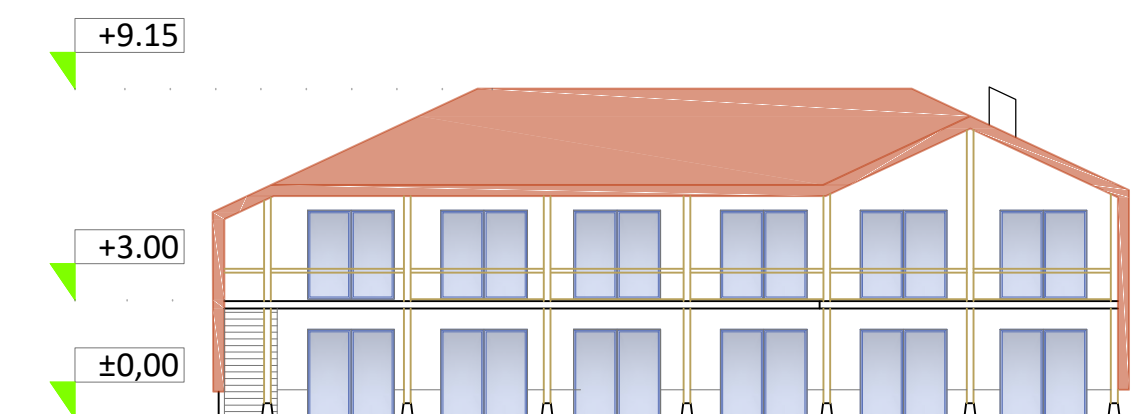
GLAVNA FASADA
