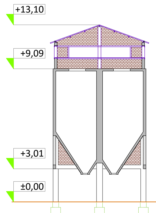
POPREČNI PRESEK
