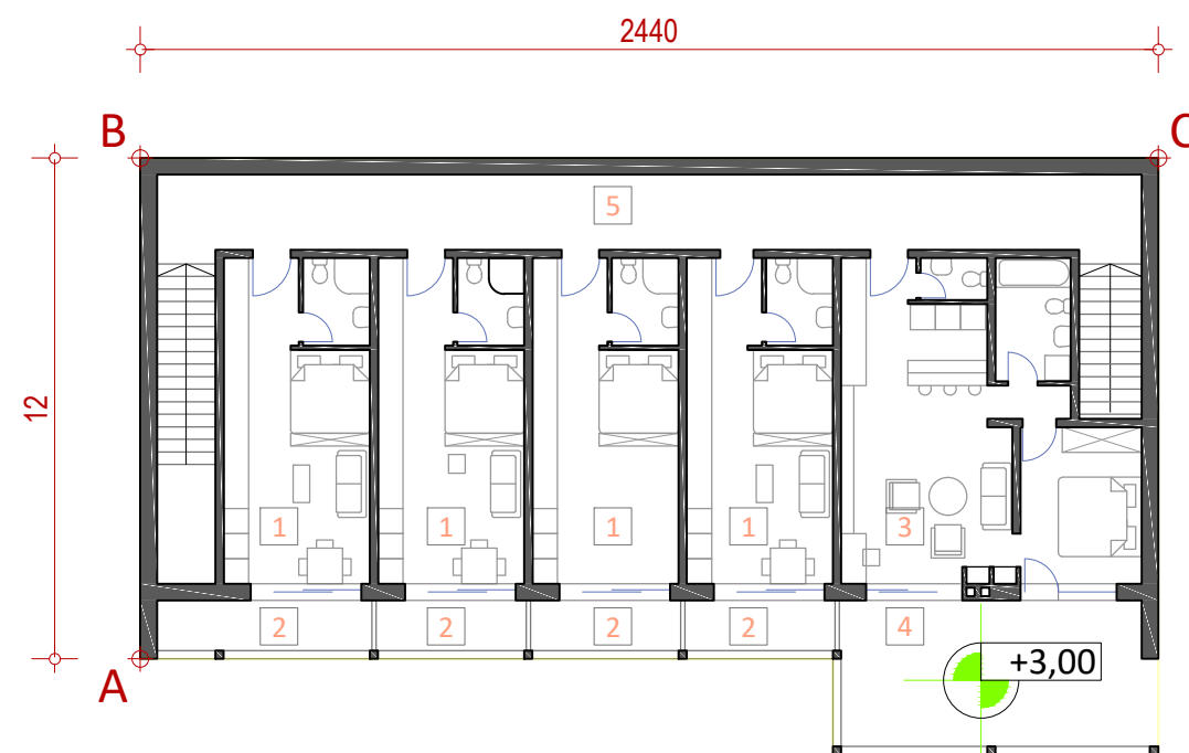
OSNOVA SPRATA
