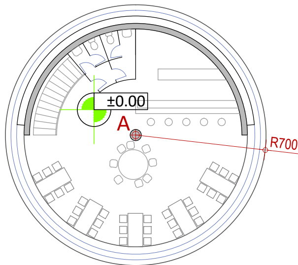
OSNOVA PRIZEMLJA
