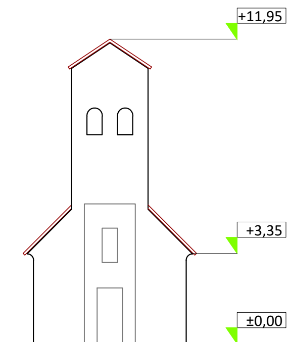
FRONTALNA FASADA
