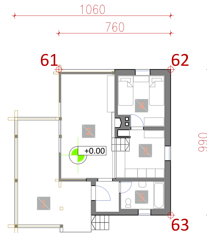
OSNOVA PRIZEMLJA
