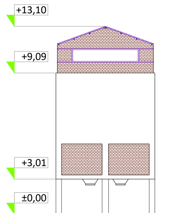
BOČNA FASADA
