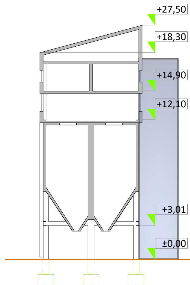
POPREČNI PRESEK
