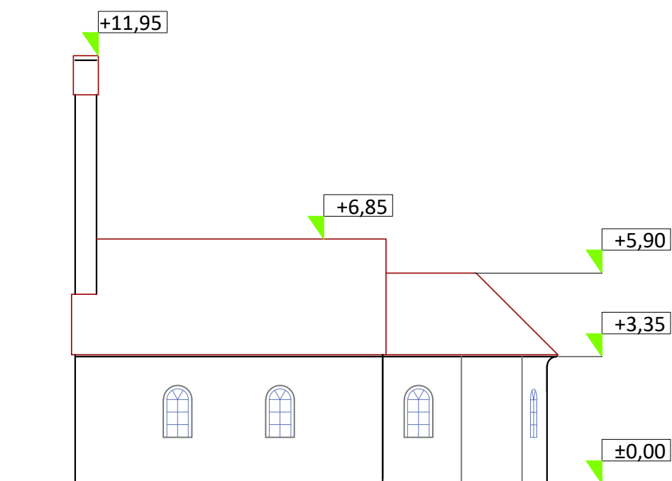
PODUŽNA FASADA
