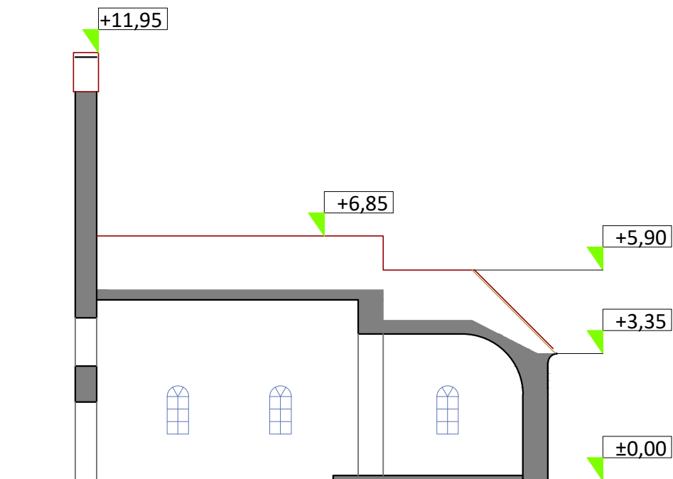
PODUŽNI PRESEK
