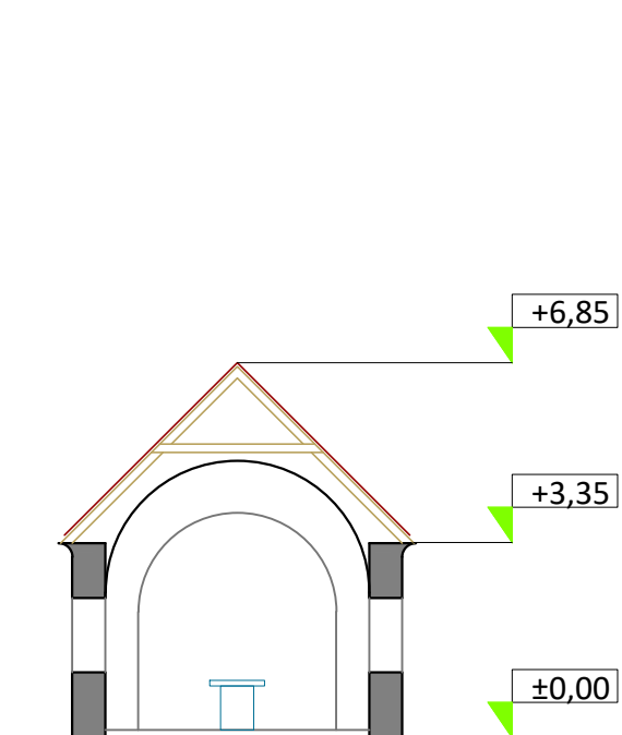
POPREČNI PRESEK
