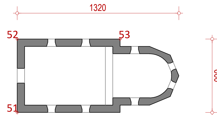
OSNOVA
