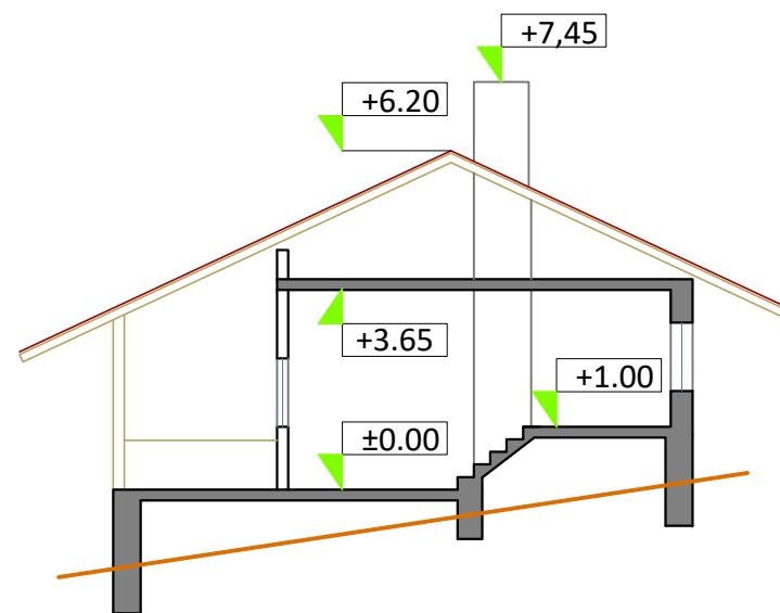
PRESEK
