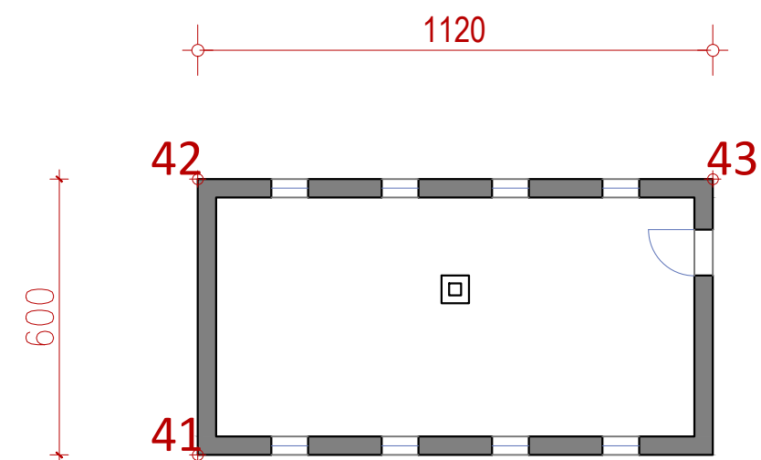
OSNOVA PRIZEMLJA
